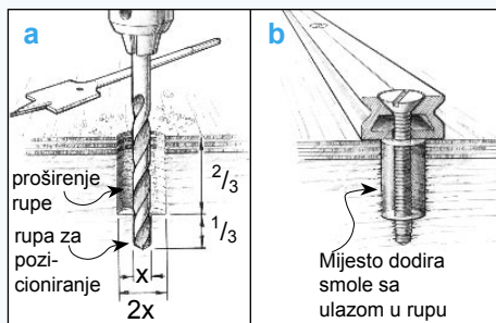
Slika 16 Izbušiti veće rupe kako bi se povećala izložena površina i količina epoksi smjese oko vijka
