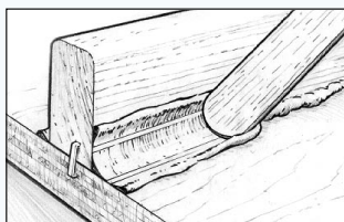
Σχήμα 13 Διαμορφώστε και εξομαλύνετε το κοίλο αρμοκάλυπτρο.
