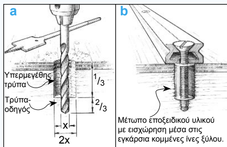
Σχήμα 16 Διανοίξετε υπερμεγέθεις τρύπες για να αυξήσετε την εκτεθειμένη επιφάνεια υποστρώματος και την ποσότητα εποξειδικού μίγματος γύρω από τη βίδα.
