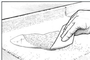
Σχήμα 29 Απλώστε το εποξειδικό μίγμα πάνω στην επιφάνεια του υφάσματος με ένα πλαστικό μάκτρο.
