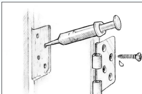
Σχήμα 15 Διαβρέξτε την εσωτερική επιφάνεια μιας κανονικού πάχους τρύπα-οδηγού και τοποθετήστε τη βίδα.
