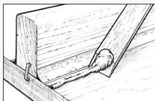
Σχήμα 14 Καθαρίστε την περίσσεια εποξειδικού μίγματος που βρίσκεται εκτός περιθωρίου.
